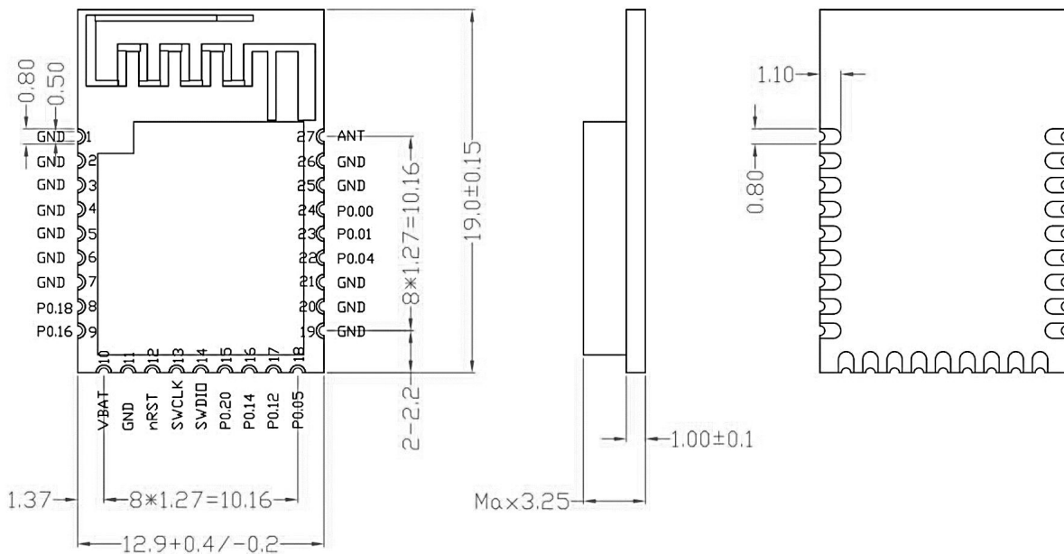
图 2- 2 E95 模组引脚布局
