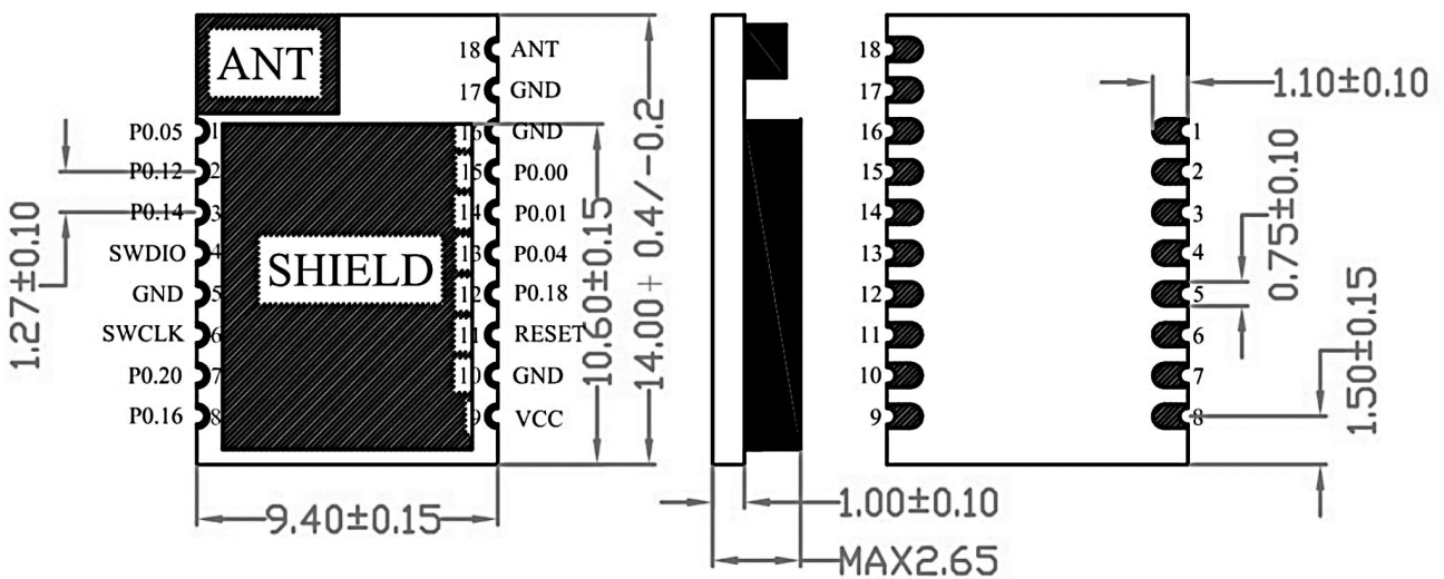
图 2- 4 S95 模组引脚布局
