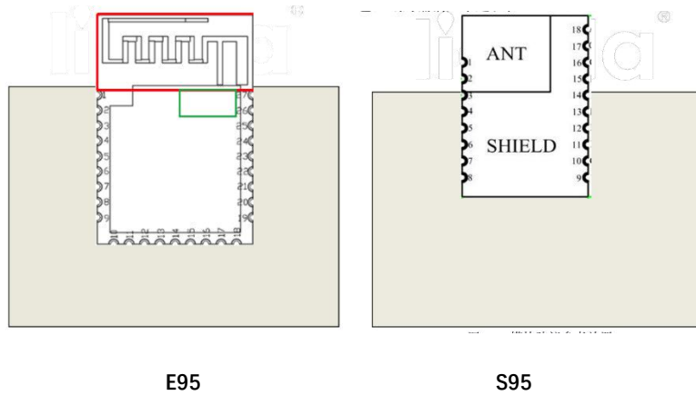
图 3- 2 Layout 规则示意图
