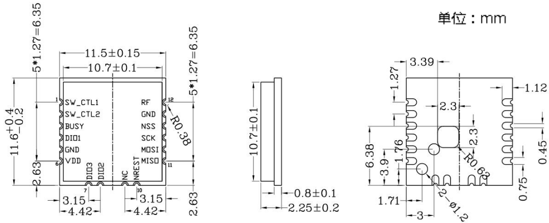
图 3-1 RL 系列模组尺寸图
