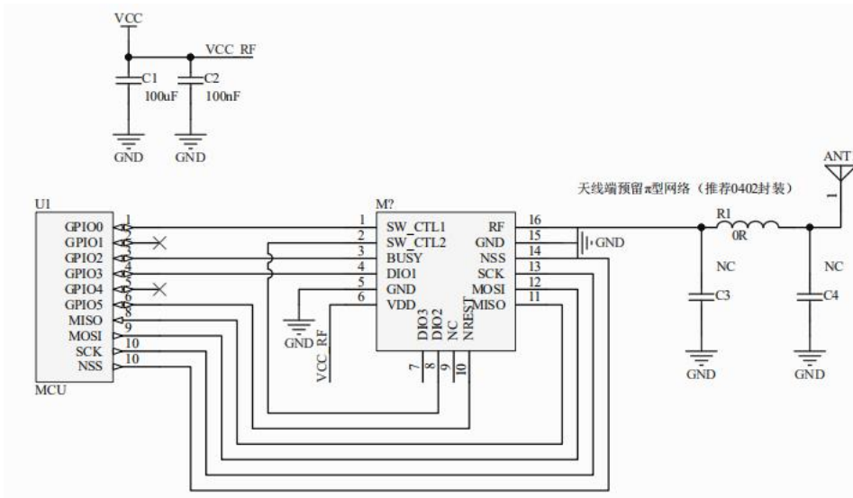
图 4-2 典型应用电路二
