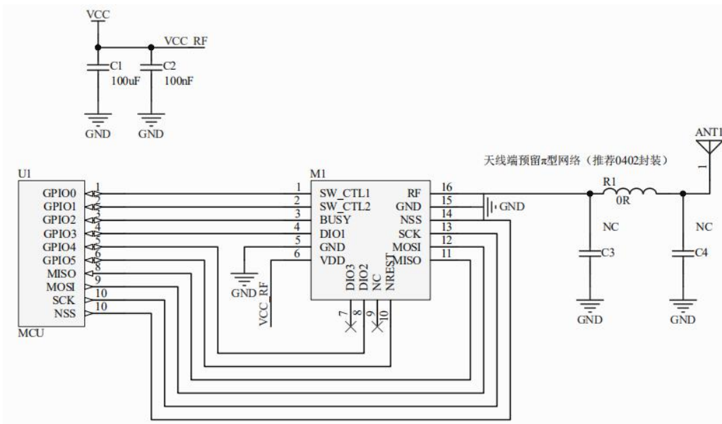
图 4-1 典型应用电路一
